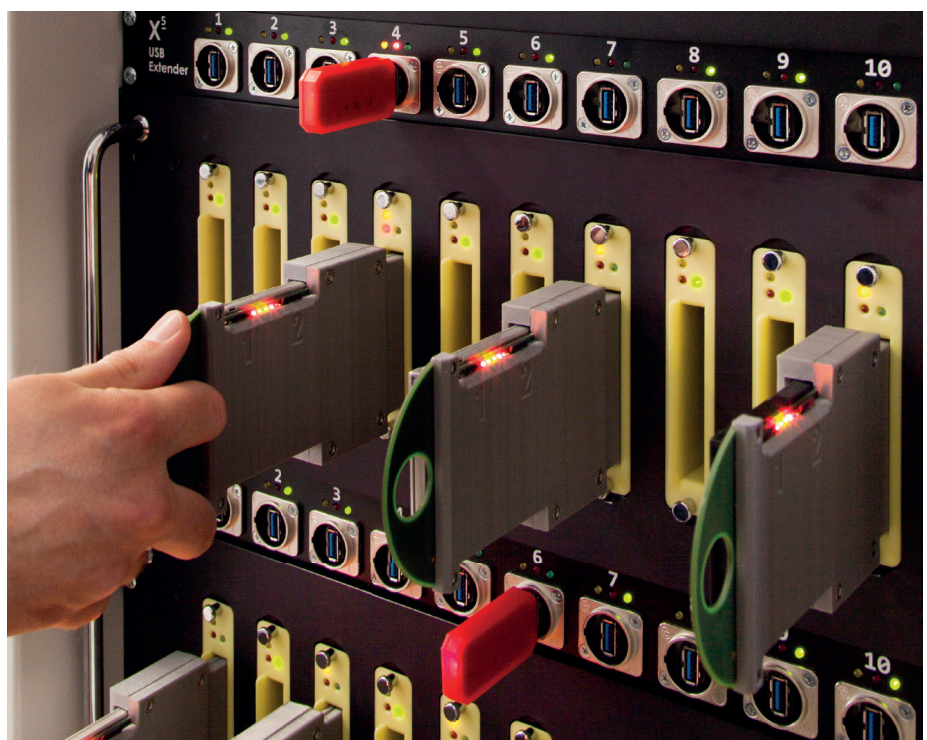
Jeder einzelne USB- und SATA-Slot ist mit LED-Anzeigen ausgestattet.
